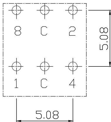
P.C.B DIMENSION
